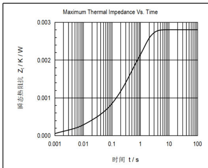
图2. 瞬态热阻抗曲线及分析公式
